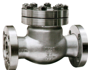
旋启式法兰止回阀
